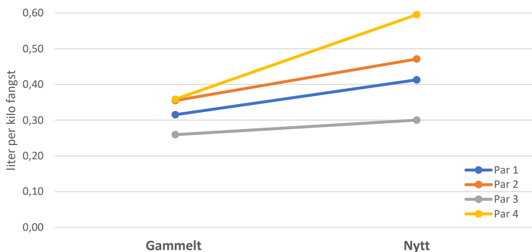
Figur 65 Gjennomsnittlig drivstofforbruk for henholdsvis gamle og nye fartøy blant fire utskiftinger i torsketrålflåten – 2012–2018 (Kilde: Fiskeridirektoratets fartøyregisteret, sluttseddeldata og Lønnsomhetsundersøkelsen)
